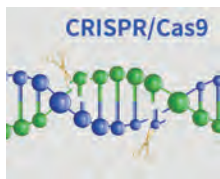
CRISPR/Cas9
