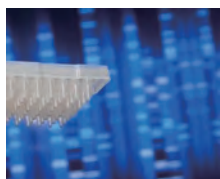
PCR
